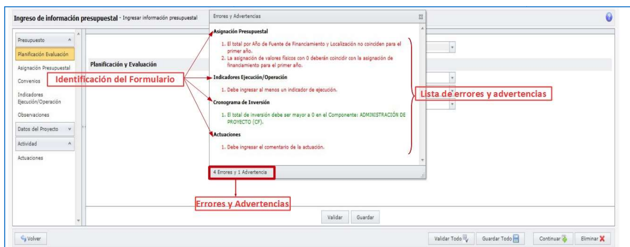
Figura 3: Errores y Advertencias
